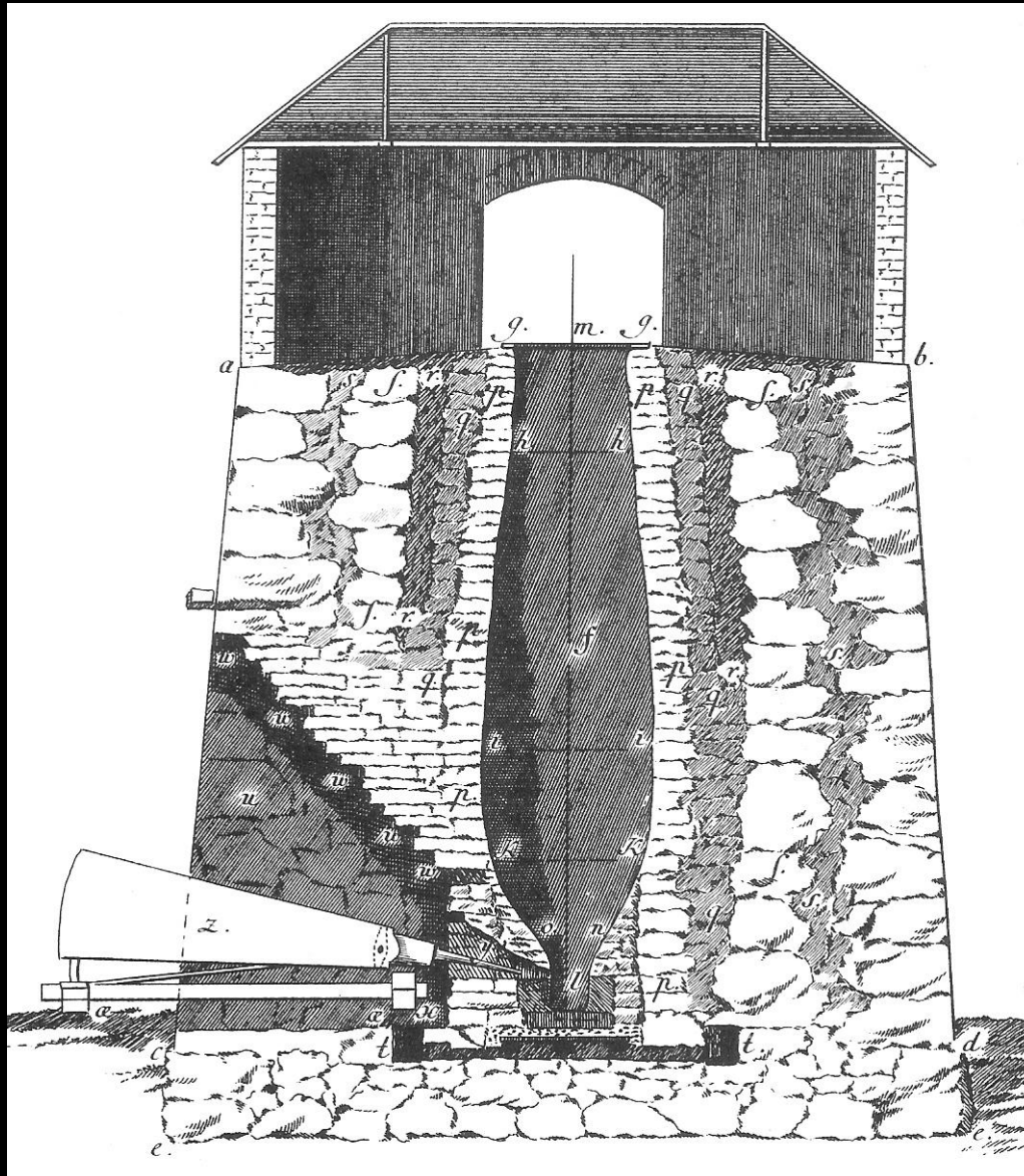
Masugnens konstruktion
